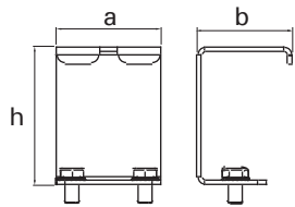
İkili Mapa Askı Takımı
