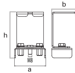
İkili Mapa ACK Kit Askı Takımı
