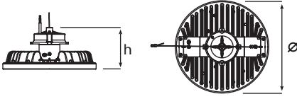
Ölçüler (mm)
