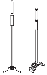
ÇUBUK-BETON ASKI TAKIMI
