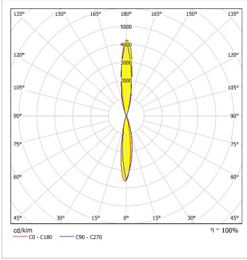
11 Derece Fotometrik Eğrisi
