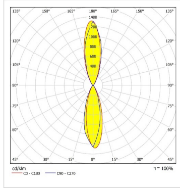
18 Derece Fotometrik Eğrisi
