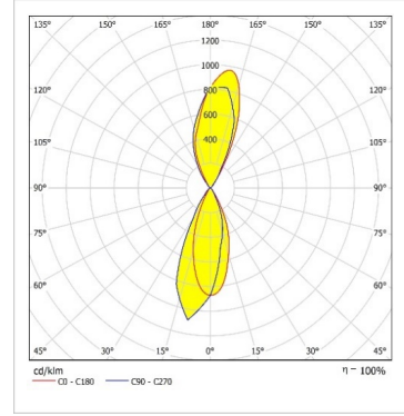
31 Derece Fotometrik Eğrisi
